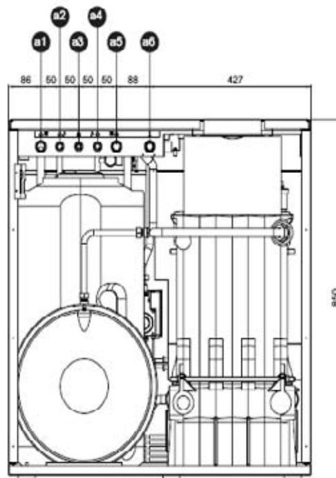
Рис. 17 – Схема подключения
