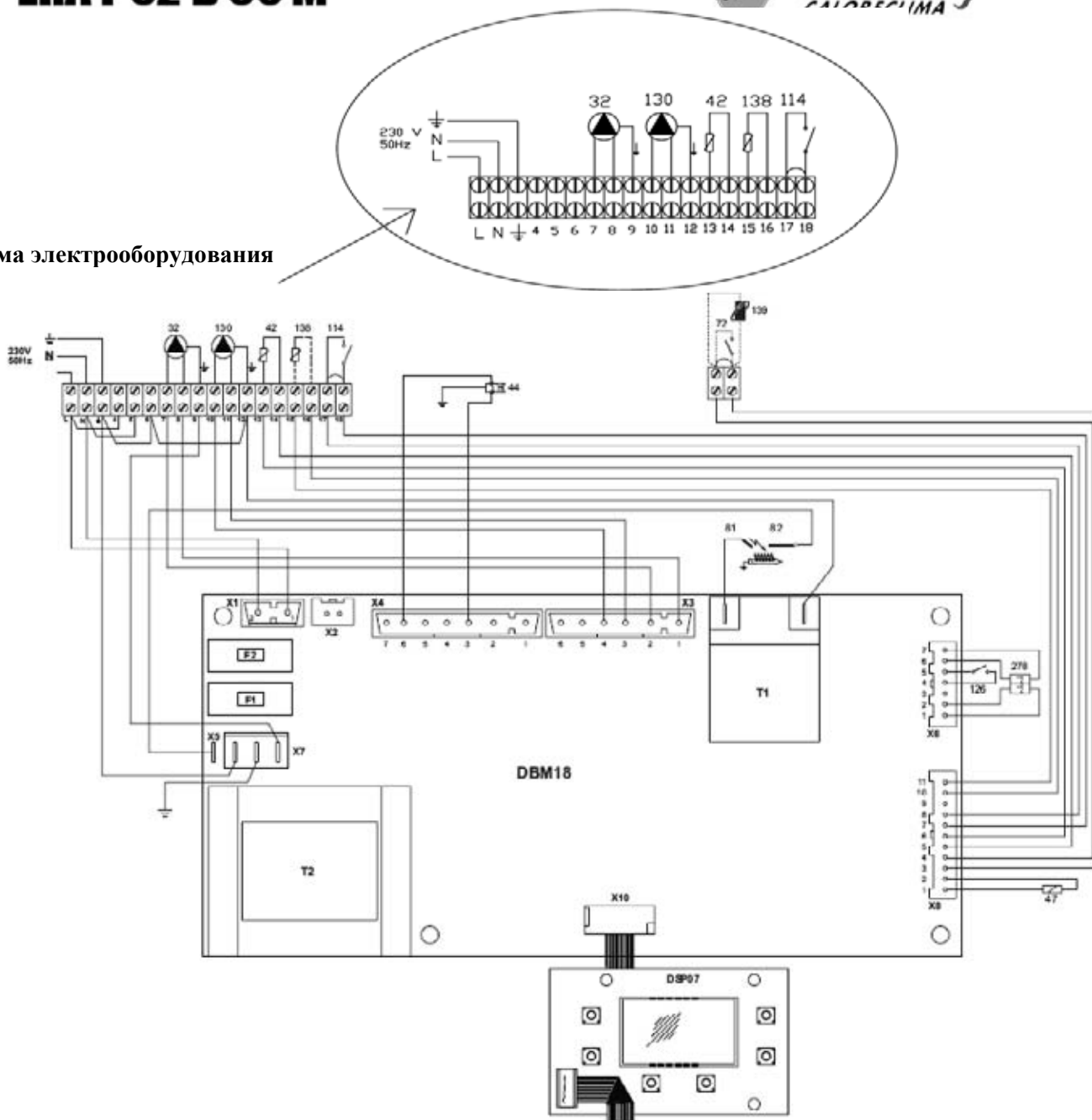
Рис. 26 – Схема электрооборудования
